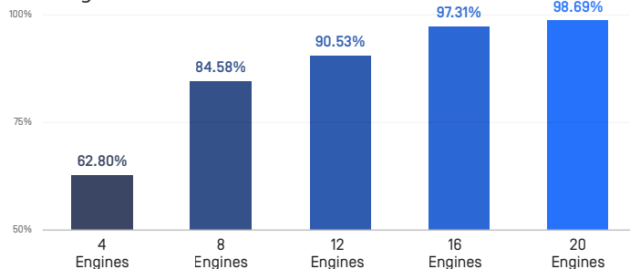
Tassi di rilevamento delle 10.000 minacce principali con OPSWAT Multi-scanning
